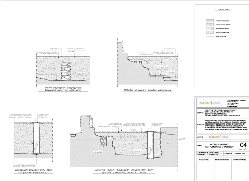
σχ.04. Κατασκευαστικές λεπτομέρειες επιχώσεων
