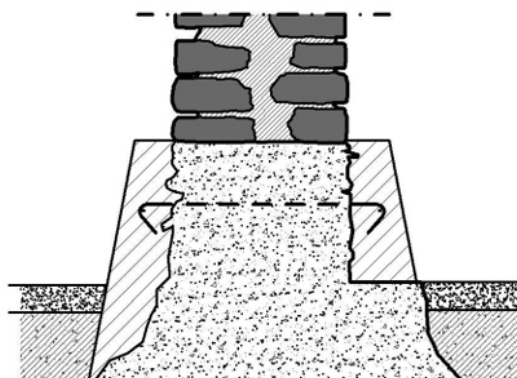
Εικόνα 1: Πλευρική αντιστήριξη με χυτά κράσπεδα
