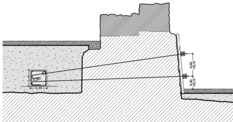
Εικόνα 3: Πλευρική αντιστήριξη εδαφικής παρειάς στον ανατολικό τοίχο του ναυδρίου
